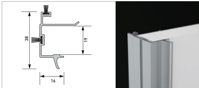
Profil vertical 560
