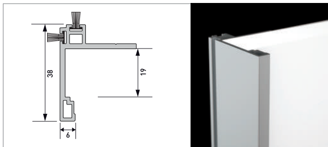
Profil vertical 510
