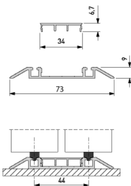
Profil vertical 2200
