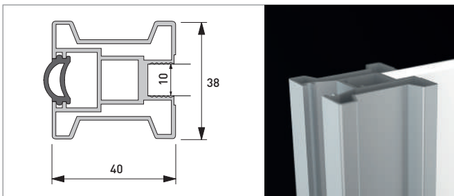
Profil vertical 1400
