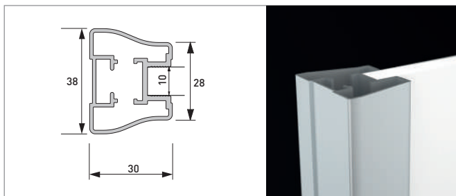
Profil vertical 1000
