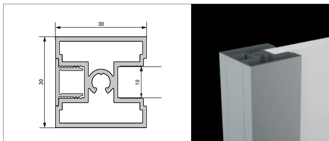
Profil vertical 3000
