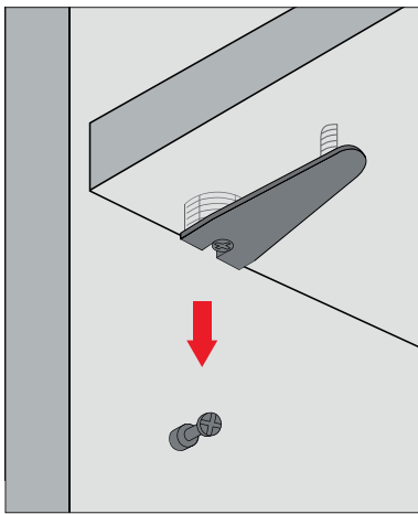
Emboîtement du plancher par le haut OU Emboîtement de la joue dans le plancher par le côté
