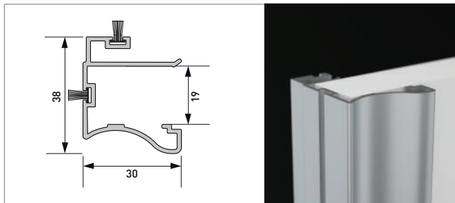
Profil vertical 500
