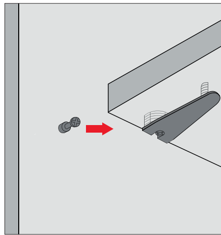
Emboîtement du plancher par le haut OU Emboîtement de la joue dans le plancher par le côté
