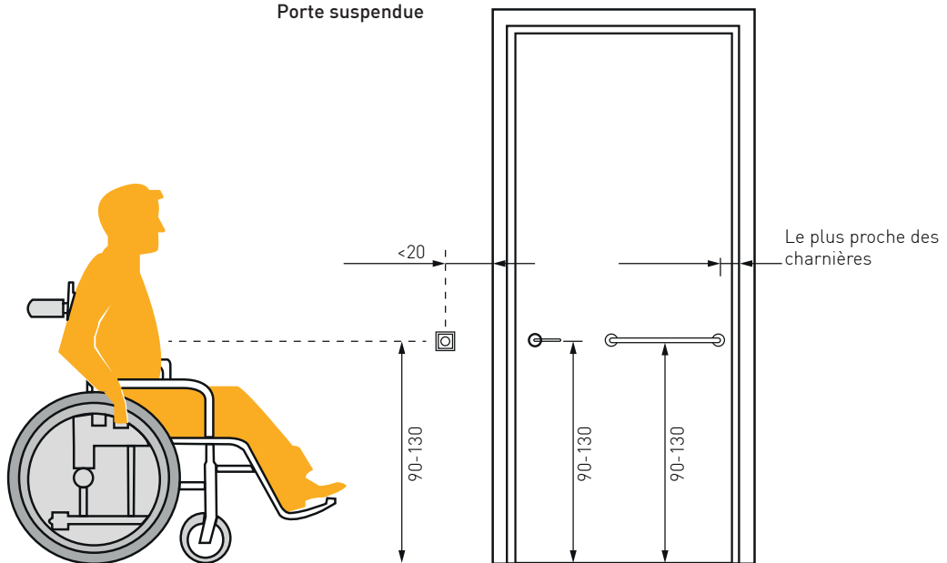
Porte suspendue
