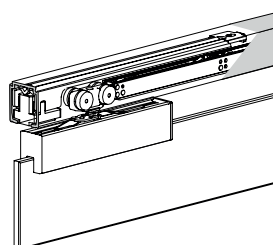
Système de suspension avec frein intégré
