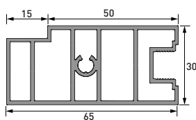
PROFIL 6500 OUVRANT
