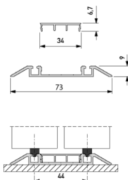
Profil vertical 1400
