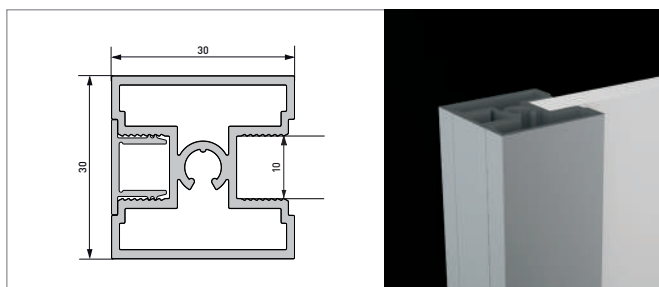
Profil vertical 3000
