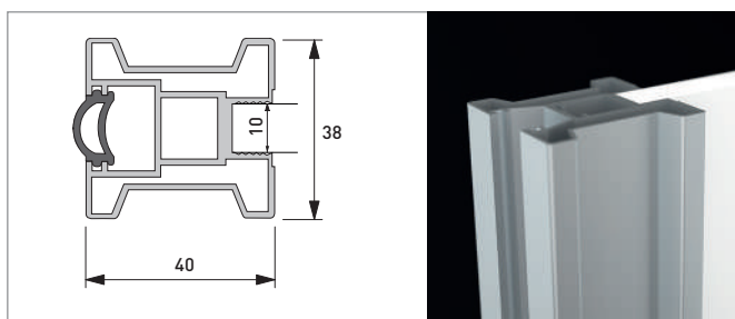
Profil vertical 1400
