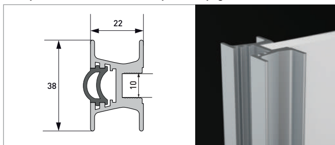
Profil vertical 2200
