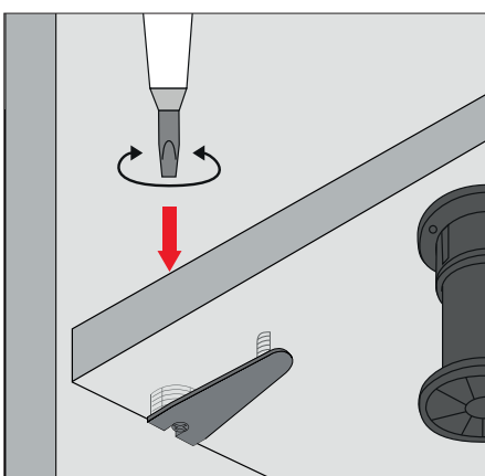
Emboîtement du plancher par le haut OU Emboîtement de la joue dans le plancher par le côté
