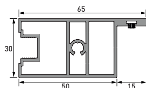
PROFIL 6501 DORMANT
