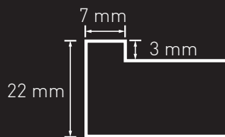
Vue de coupe
